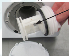
Фильтр насоса
